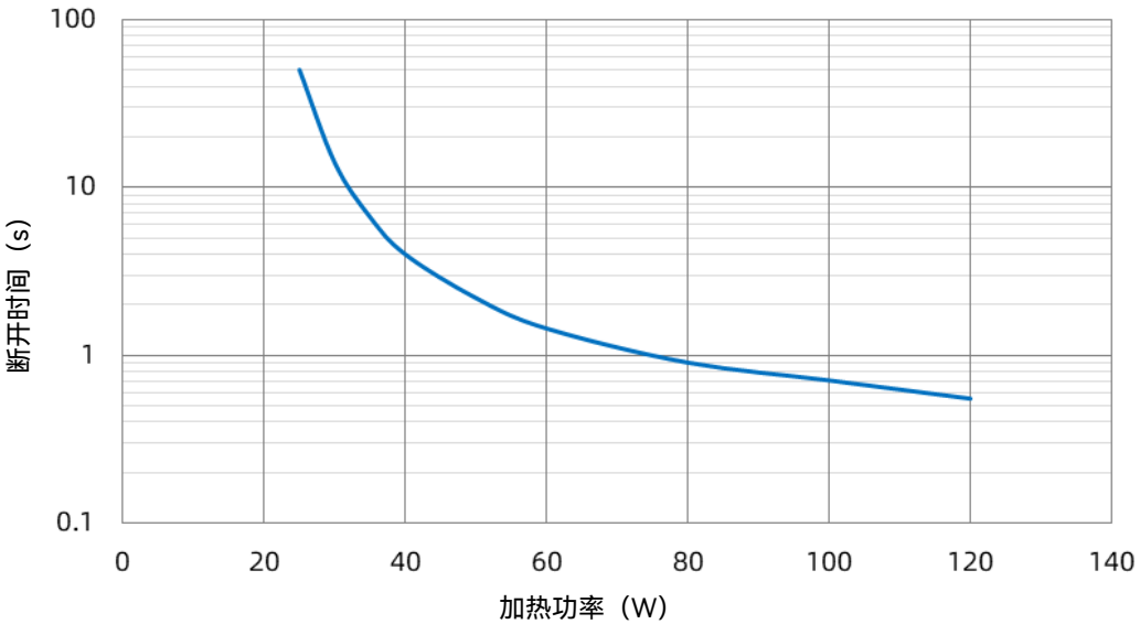
SHP 75 A 功率-时间曲线
