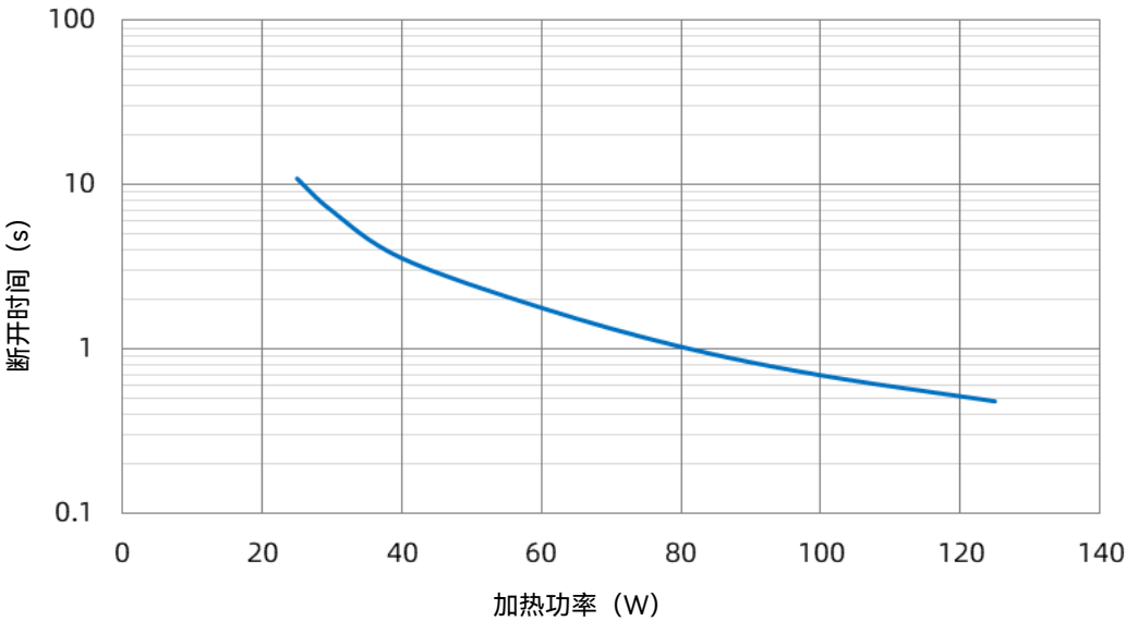
SHP 60 A 功率-时间曲线
