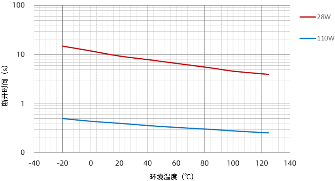
SHP 60 A 功率-温度曲线
