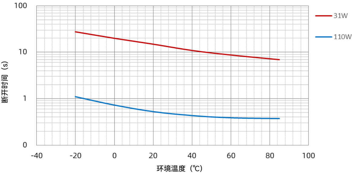
SHP 75 A 功率-温度曲线
